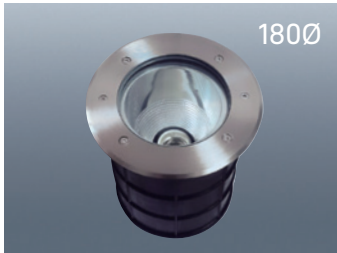
UG30 사이즈 W180×H210 전 압 AC220V 램 프 E-26 BASE / LED PAR30 램프등
