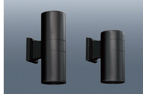
BL30 1등, 2등 (흑색) 사이즈 W110×H200 1등 / W110×H300 2등 전 력 PAR-30, LED PAR-30용
