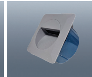
계단310 사이즈 W125×H125 전 압 AC220V 전 력 2.5W 빛색상 전구색
