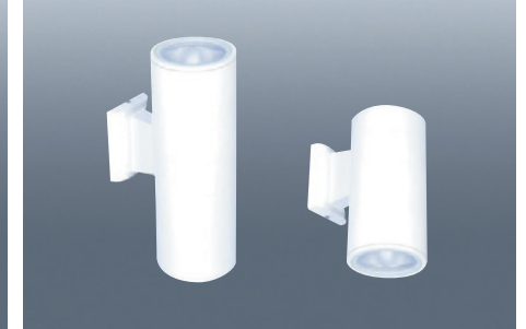
BL30 1등, 2등 (화이트) 사이즈 W110×H200 1등 / W110×H300 2등 전 력 PAR-30, LED PAR-30용
