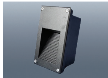
LED계단매입 세로 블랙 사이즈 W98×D162×H80 전 압 AC220V 전 력 5W 빛색상 전구색/주광색/4000K
