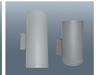
BL150 1등, 2등 (회색) 사이즈 W200×H350 1등 W200×H515 2등 전 력 HQI-70W 150W, CDM-T 70W 150W용
