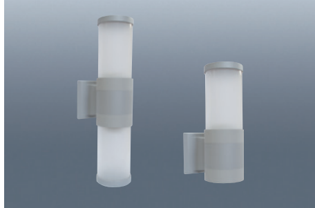
BL 20 1등, 2등 사이즈 W90×H205 1등 / W90×H270 2등 전 력 EL램프, LED 벌브용
