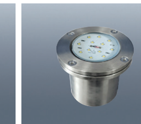
WP50N 확산형 사이즈 W90×H70 전 압 DC12V / DC24V 전 력 3W~6W 빛색상 전구/주광/적/청/녹/RGB
