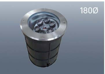
UG30 집중형 각도 사이즈 W180×H210 전 압 AC220V / DC12V 전 력 6W~10W 빛색상 전구/주광/적/청/녹/4000K등
