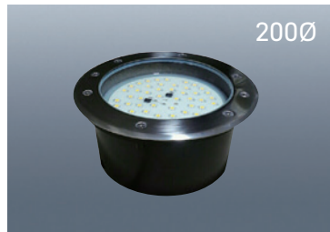
UG200WJ 확산형 사이즈 W200×H89 전 압 AC220V / DC12V 전 력 20W~25W 빛색상 전구색/주광색
