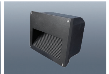
WL18FPL 블랙 사이즈 W230×D195×H115 전 압 AC220V 전 력 6.5W / 8.7W / 12W 빛색상 전구색/주광색/4000K
