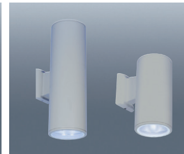
BLS30 1등, 2등 (회색) 사이즈 W120×H210 1등 W120×H310 2등 전 력 PAR-30, LED PAR-30용
