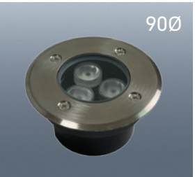
UG90WJ 사이즈 W90×H40 전 압 AC220V 전 력 3W 빛색상 전구색
