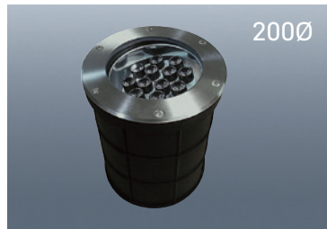
UG38ST 집종형 각도 사이즈 W200×H225 전 압 AC220V / DC12V / DC24V 전 력 12W~15W 빛색상 전구/주광/적/청/녹/RGB/4000K등
