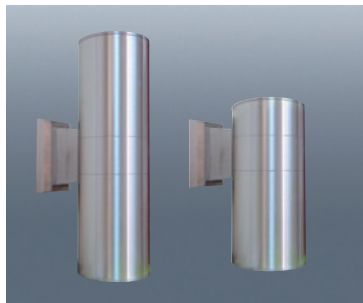
BL30 1등, 2등 (샤틴/동도금) 사이즈 W110×H200 1등 W110×H300 2등 전 력 PAR-30, LED PAR-30용
