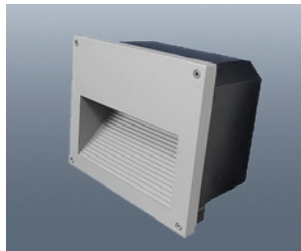
WL18FPL 그레이 사이즈 W230×D195×H115 전 압 AC220V 전 력 6.5W / 8.7W / 12W 빛색상 전구색/주광색/4000K
