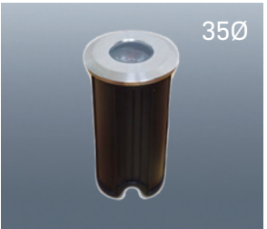
UG50-35 사이즈 W35×H61 전 압 DC12V 전 력 1.5W 빛색상 전구색
