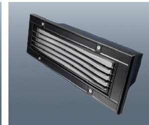
계단창살창 사이즈 W305×D112×H90 전 압 AC220V 전 력 6W / 9W 빛색상 전구색/주광색/4000K
