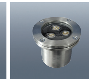
WP50N 집종형 사이즈 W90×H70 전 압 DC12V 전 력 3W 빛색상 전구/주광/적/청/녹/4000K등
