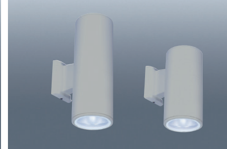
BL30 1등, 2등 (회색) 사이즈 W110×H200 1등 / W110×H300 2등 전 력 PAR-30, LED PAR-30용
