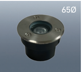
UG65WJ 사이즈 W65×H40 전 압 AC220V 전 력 1W 빛색상 전구색
