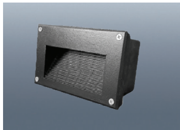
LED계단매입 가로 블랙 사이즈 W162×D98×H80 전 압 AC220V 전 력 5W 빛색상 전구색/주광색/4000K
