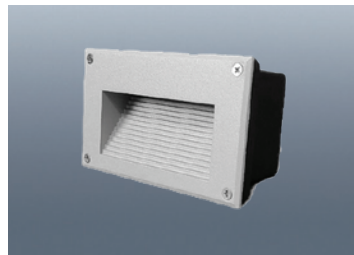
LED계단매입 가로 그레이 사이즈 W162×D98×H80 전 압 AC220V 전 력 5W 빛색상 전구색/주광색/4000K
