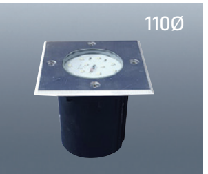
UG50S 확산형 사이즈 W85×H117 전 압 AC220V / DC12V / DC24V 전 력 3W / 6W 빛색상 전구/주광/적/청/녹/RGB/4000K등
