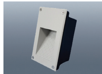
LED계단매입 세로 그레이 사이즈 W98×D162×H80 전 압 AC220V 전 력 5W 빛색상 전구색/주광색/4000K
